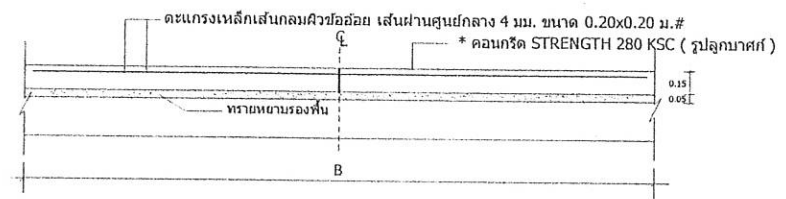
รูปตัดถนนคอนกรีตเสริมเหล็ก ก/ก NOT TO SCALE
